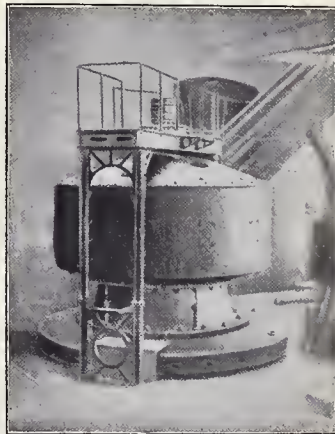
Una delle dinamo di 5000 cavalli dell'impianto del Niagara.
